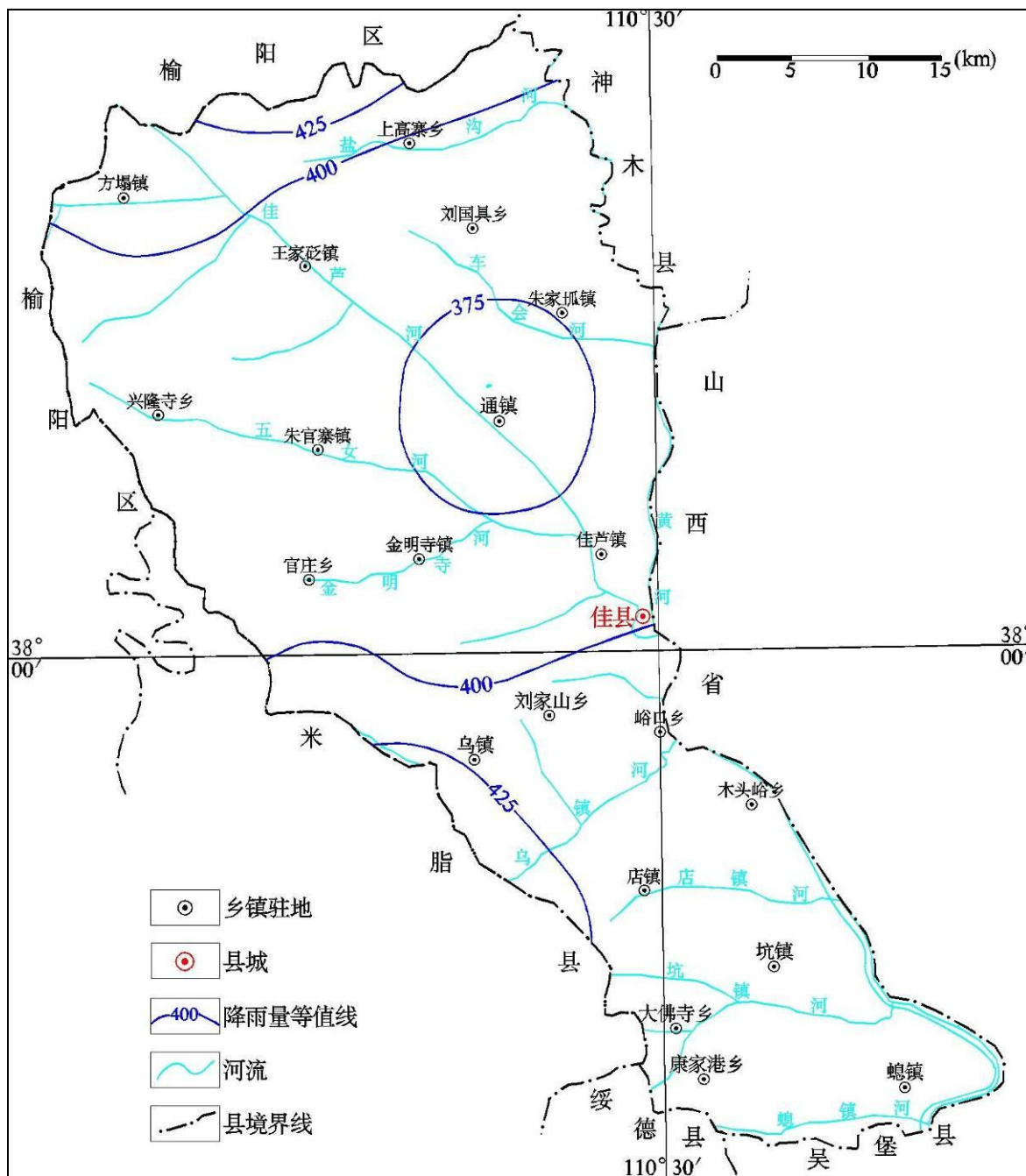
图 1-6 佳县年降雨量等值线图
